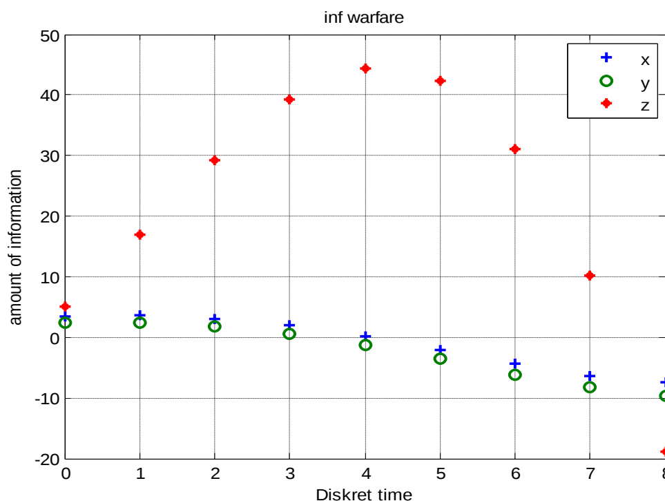
ნახატი 2.2.14 მხარეთა აქტიურობის გრაფიკები: დისკრეტული, D < 0 , პირველი მხარის სასტარტო პირობა მეტია მეორისაზე, ფუძე ერთზე ნაკლებია p < 1 D = \alpha^2 - 8\beta\gamma < 0 \alpha = 0,1 ; \beta = 0,05 ; \gamma = 2 x_0 > y_0 x_0 = 3.5 > y_0 = 2.5 z_0 = 5
