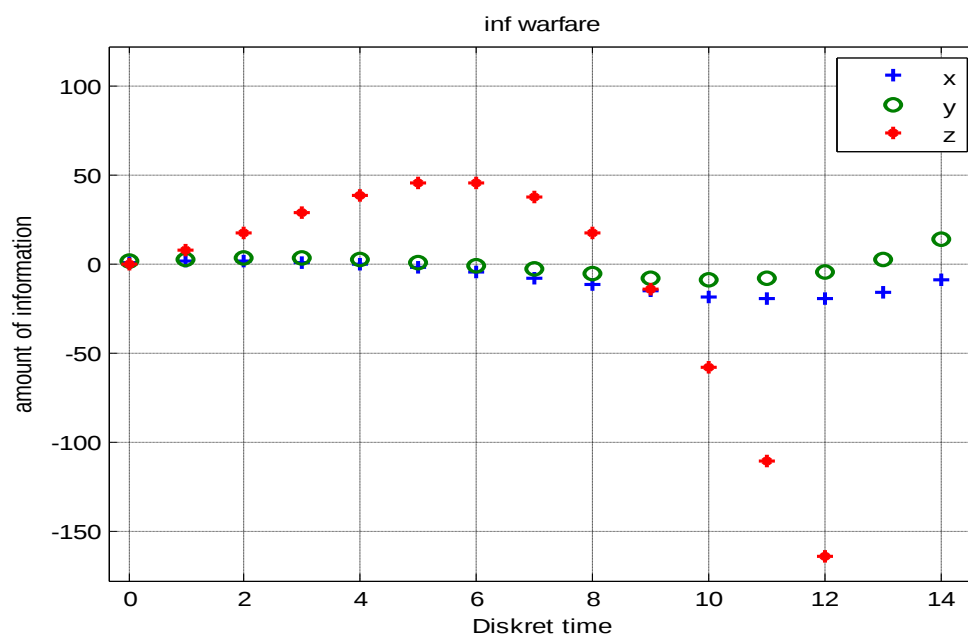
ნახატი 2.1.15. მხარეთა აქტიურობის გრაფიკები: D < 0 , მეორის სასტარტო პირობა მეტია პირველზე და ფუძე ერთზე მეტია p > 1 , ალფა მარცხენა ზღვართანაა ახლოს (0,1708) D = \alpha^2 - 8\beta\gamma < 0 \alpha = 0,25 ; \beta = 0,05 ; \gamma = 2 x_0 < y_0 x_0 = 1.5 y_0 = 2.5
