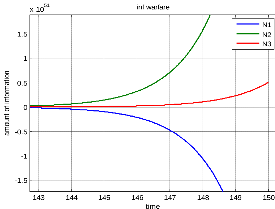
ნახატი 1.2.3. მხარეთა აქტიურობის გრაფიკები: D > 0 , მეორის სასტარტო პირობა მეტია პირველზე D = \alpha^2 - 8\beta\gamma > 0 \alpha = 0,8 ; \beta = 0,05 ; \gamma = 0,16 ; N_{10} = 1,5 N_{20} = 2,5
