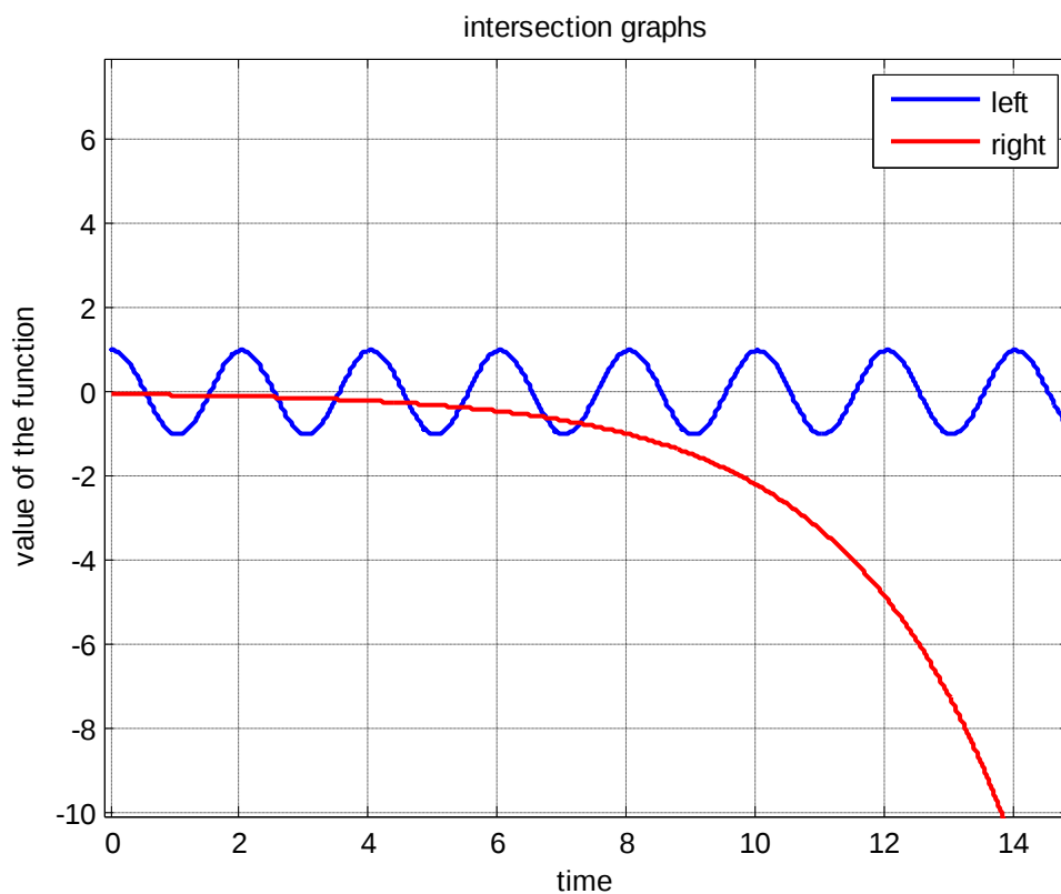
ნახატი 1.2.6. (1.2.56) განტოლების ამოხსნის გრაფიკული ხერხი, \gamma=100
